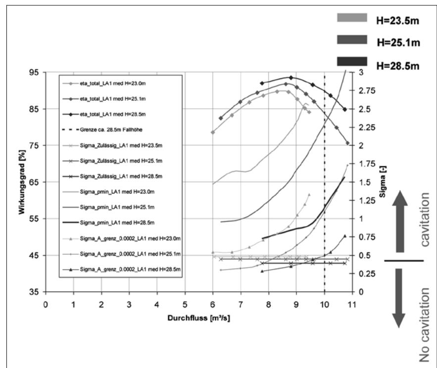
Bild 7: Verlauf der Thoma-Zahl einer Francis-Turbine und Vergleich mit den Anlagewerten für verschiedenen Leitschaufelstellungen und Fallhöhen
